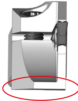
Simulationsanalyse Abdrängungswert: 0.013 mm
