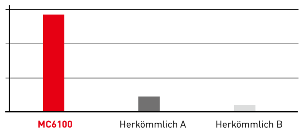
Das Verhältnis von \text{Al}_2\text{O}_3 -Kristallkörnern mit gleicher Ausrichtung.
