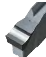
GL Spanbrecher (Für Aluminiumlegierungen)
